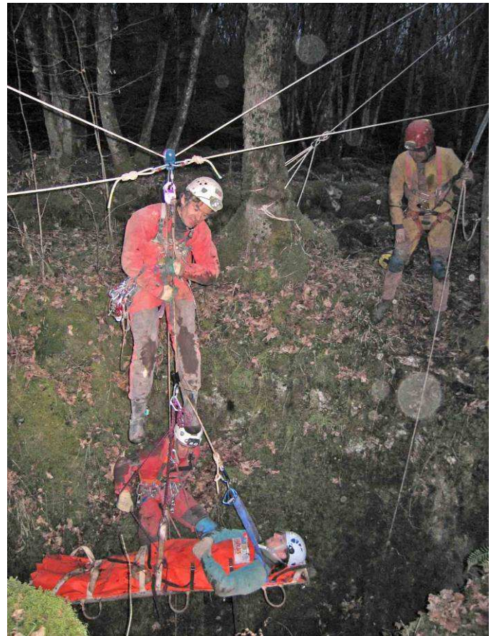
Mis en œuvre d'un balancier sur tyrolienne
